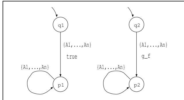
Fig. 26. CoNP constraint automata
