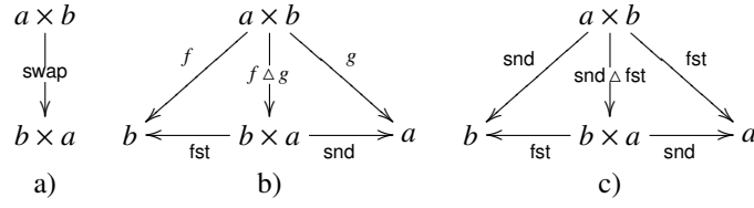
Figura 3.1: Derivação do swap usando diagramas.
