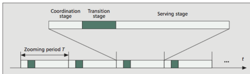
Figura 2.9: Processo dos algoritmos de cell zooming . Source: [14].
