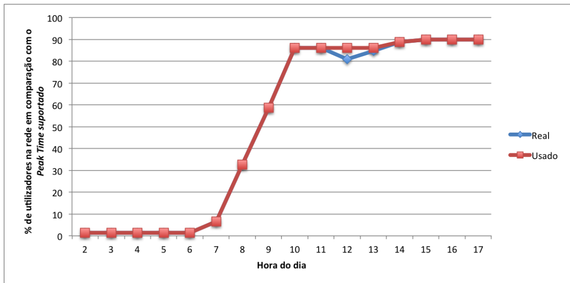
Figura 3.16: Comparação entre os valores reais e os valores utilizados na simulação do Tráfego 5.
