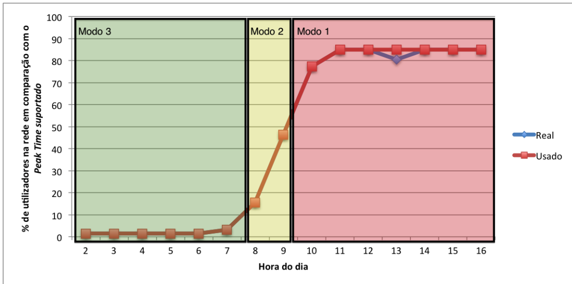
Figura 4.4: Tempo de funcionamento em cada modo no Tráfego 4.
