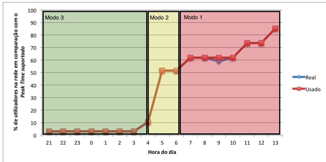
Figura 4.3: Tempo de funcionamento em cada modo no Tráfego 3.
