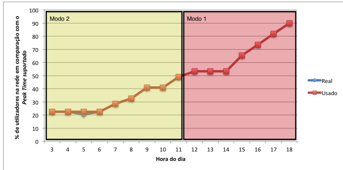
Figura 4.16: Tempo de funcionamento em cada modo no Tráfego 1 com o threshold de 5%.
