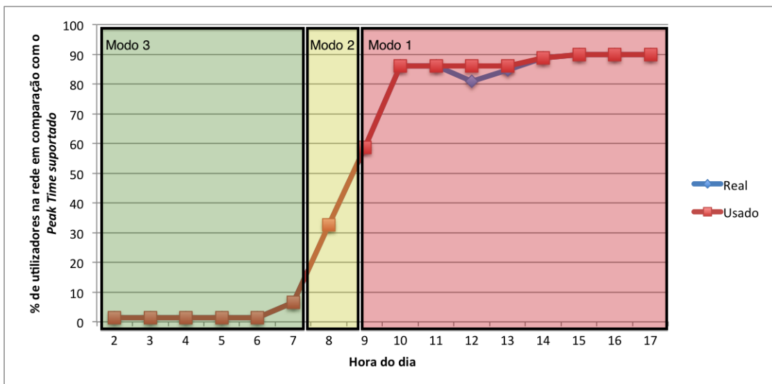
Figura 4.5: Tempo de funcionamento em cada modo no Tráfego 5.
