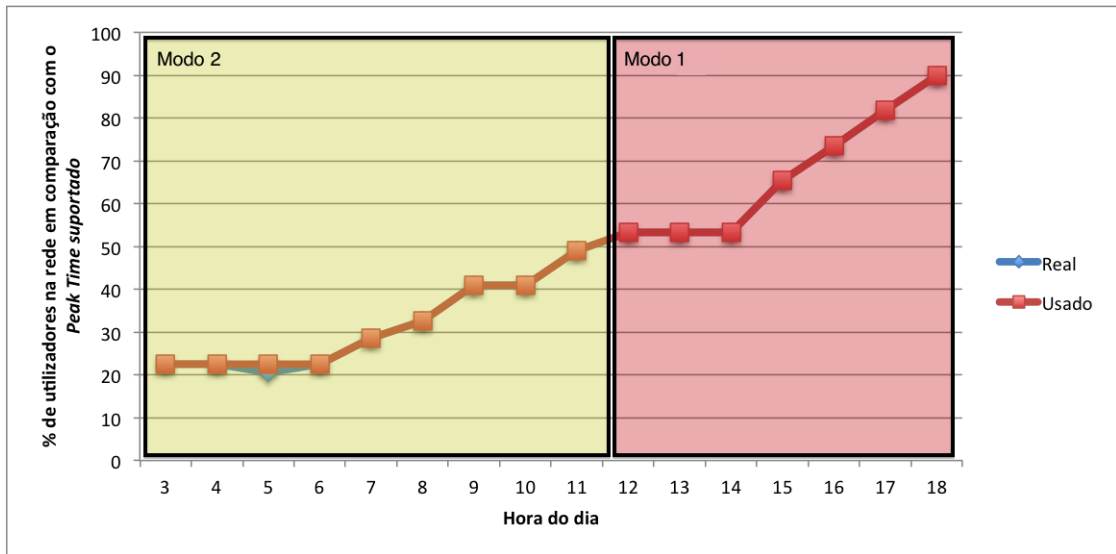
Figura 4.11: Tempo de funcionamento em cada modo no Tráfego 1 com o threshold de 5%.
