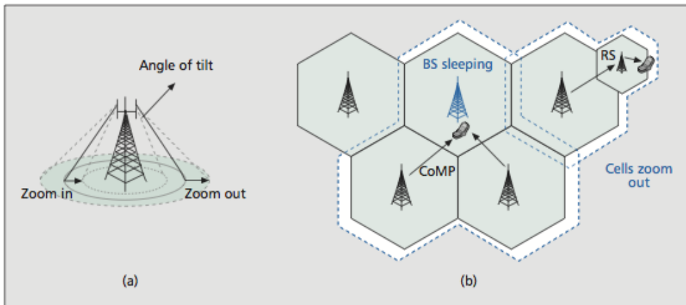
Figura 2.8: Técnicas para implementar cell zooming : a) 'aumento' ou 'diminuição' das células com ajustamento dos parâmetros físicos das mesmas; b) 'aumento' ou 'diminuição' das células através de cooperação entre estações base e retransmissão. Source: [14].
