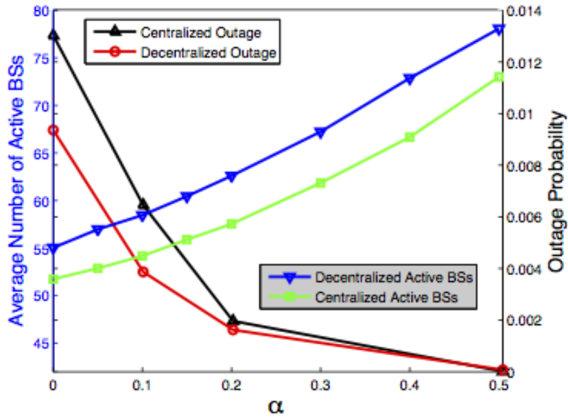
Figura 2.12: Desempenho do algoritmo. Source: [16].
