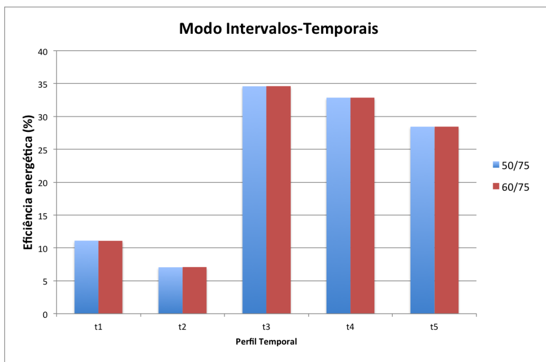
Figura 4.23: Comparação da eficiência energética nos diferentes perfis no Modo Intervalos-Temporais entre o tipo de capacidade 50/75 e 60/75.
