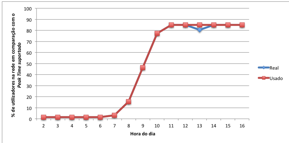
Figura 3.15: Comparação entre os valores reais e os valores utilizados na simulação do Tráfego 4.
