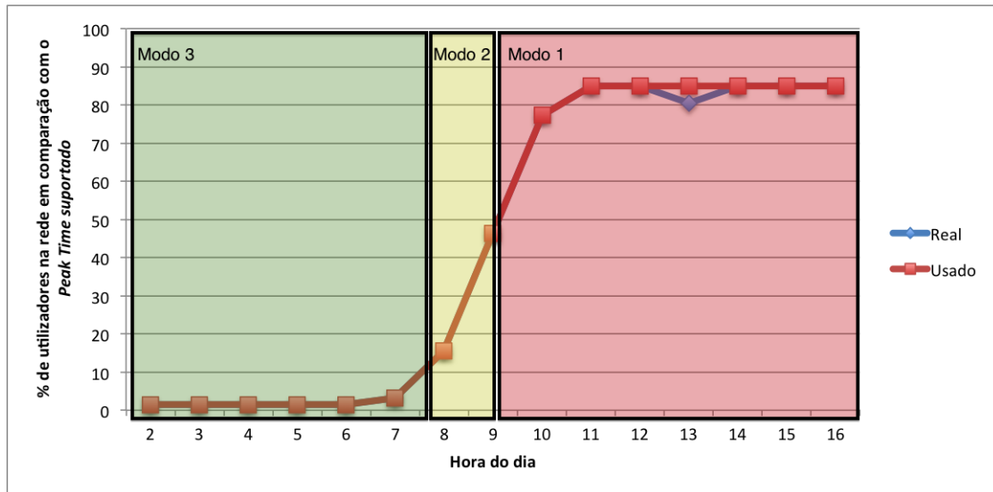
Figura 4.14: Tempo de funcionamento em cada modo no Tráfego 4 com o threshold de 15%.
