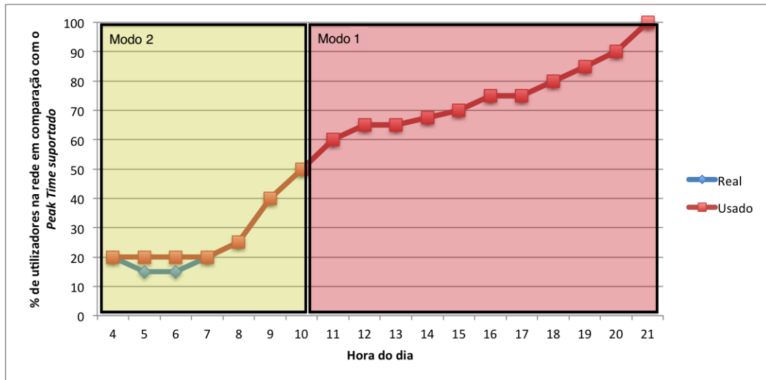
Figura 4.7: Tempo de funcionamento em cada modo no Tráfego 2.
