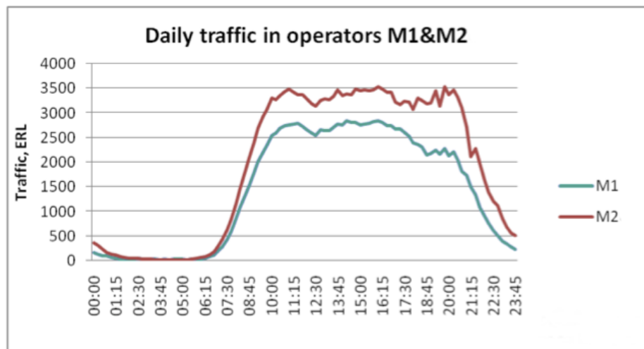
Figura 3.10: Perfis de tráfego diários (Segunda). Source: [25]
