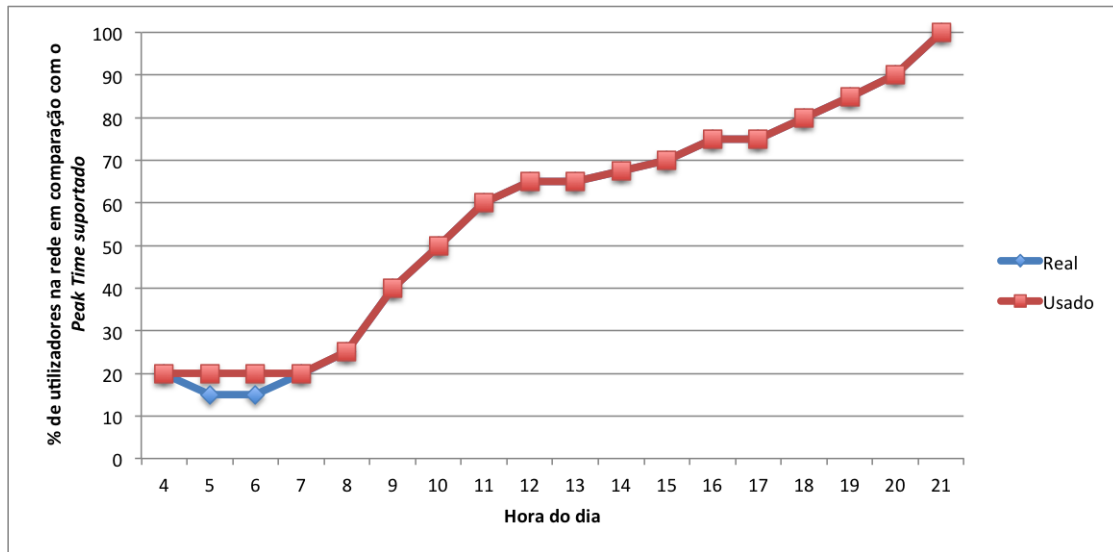
Figura 3.13: Comparação entre os valores reais e os valores utilizados na simulação do Tráfego 2.
