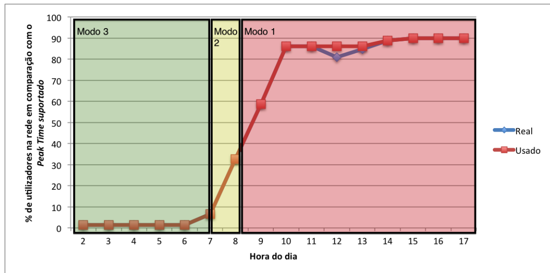
Figura 4.20: Tempo de funcionamento em cada modo no Tráfego 5 com o threshold de 35%.
