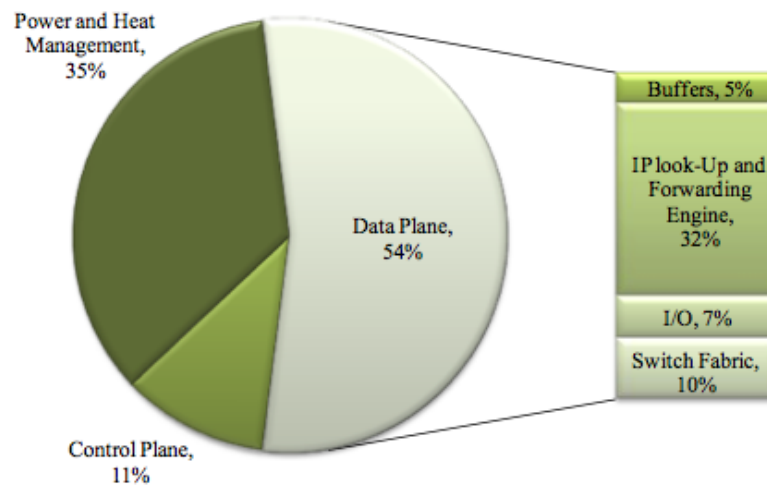
Figura 2.3: Estimativa das fontes do consumo de energia nos routers IP de gama alta. Source: [11].
