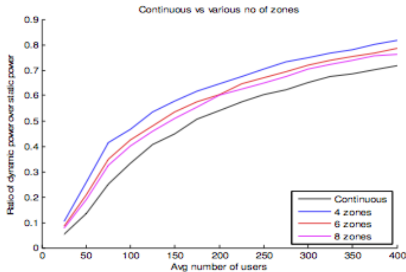
Figura 2.15: Rácio entre a energia consumida no modo dinâmico sobre o estático para diferentes valores no número de zonas discretas Z . Source: [18].
