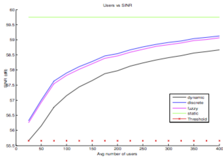
Figura 2.18: Média do SINR recebido com e sem cell zooming em função do número de utilizadores. Source: [18].
