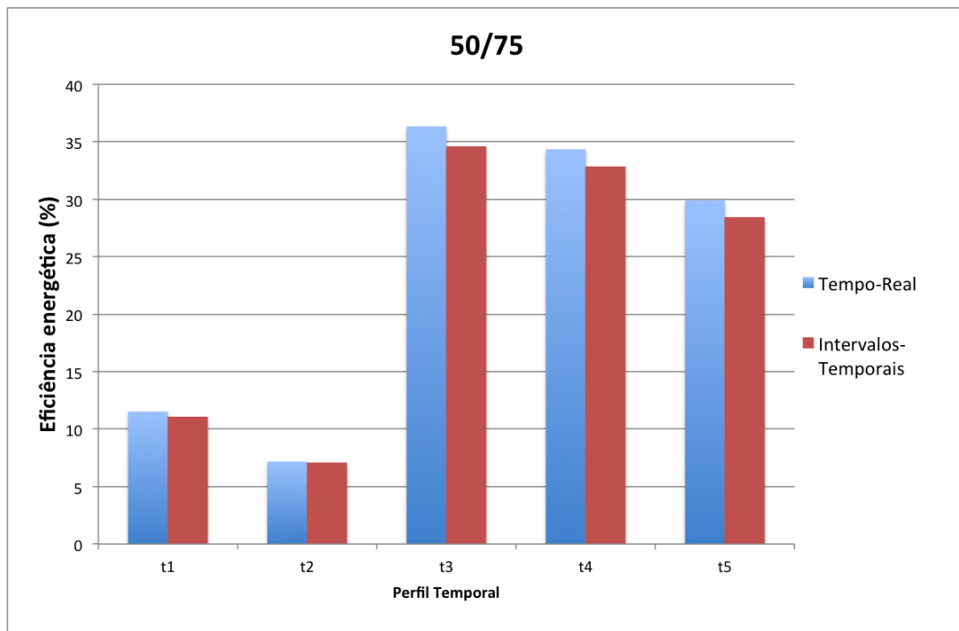
Figura 4.22: Comparação da eficiência energético nos diferentes perfis no Modo Tempo-Real e Intervalos-Temporais para o tipo de capacidade 50/75.
