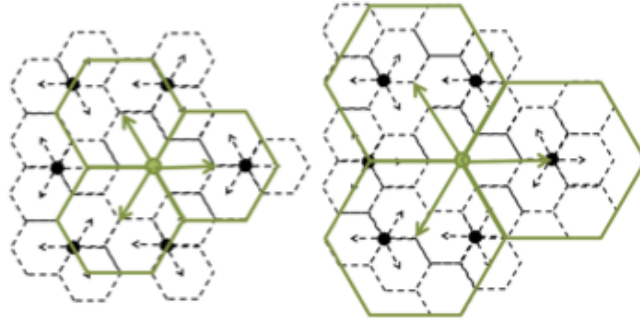
Figura 3.2: Configuração em hexágono tri-sectorial: 3 células desligadas em 4 ou 8 em 9. Source: [21].
