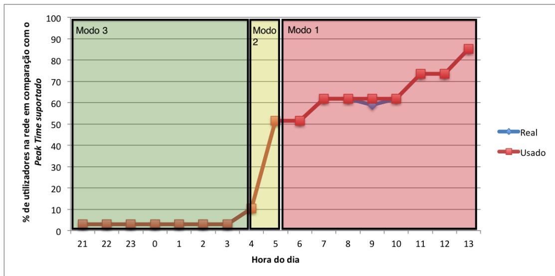
Figura 4.8: Tempo de funcionamento em cada modo no Tráfego 3.
