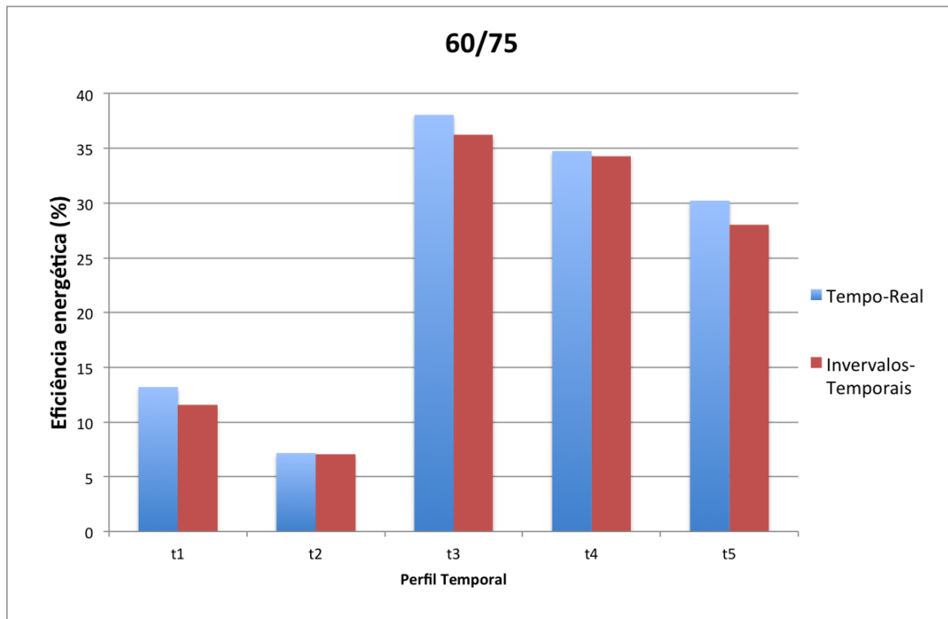
Figura 4.21: Comparação da eficiência energética nos diferentes perfis no Modo Tempo-Real e Intervalos-Temporais para o tipo de capacidade 60/75.
