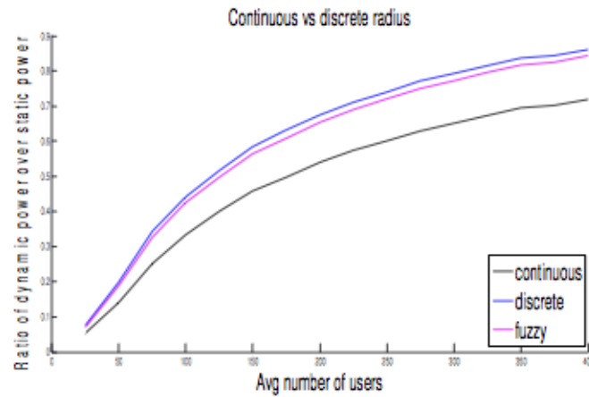
Figura 2.17: Rácio entre a energia consumida no modo dinâmico sobre o estático para os algoritmos continuous , discrete e fuzzy . Source: [18].
