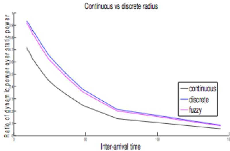
Figura 2.16: Rácio entre a energia consumida no modo dinâmico sobre o estático vs média entre intervalos de chegada de pacotes . Source: [18].
