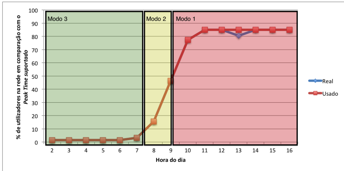
Figura 4.19: Tempo de funcionamento em cada modo no Tráfego 4 com o threshold de 30%.
